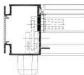
MANŒUVRE PAR TREUIL
