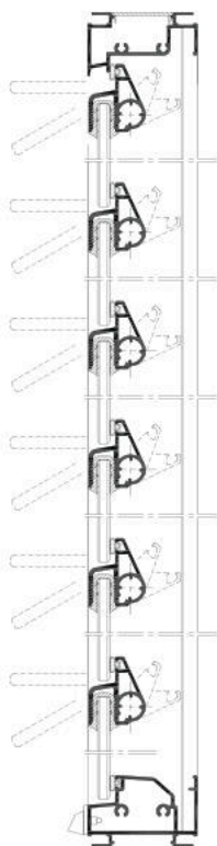
CHÂSSIS STANDARD
