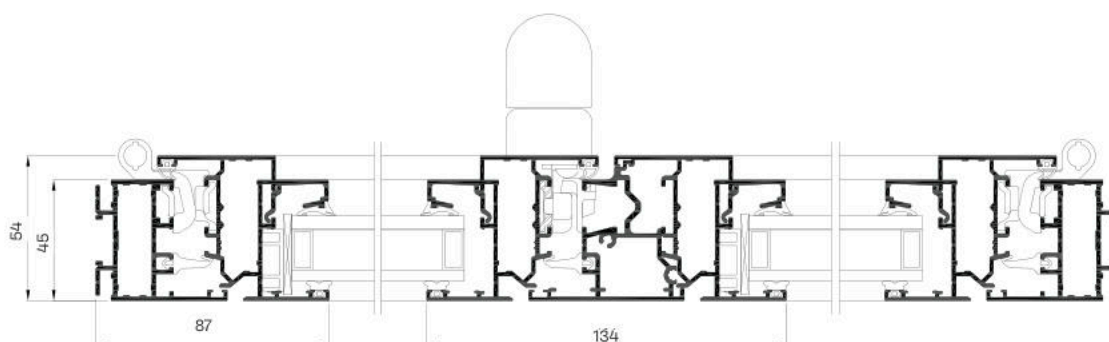
FENÊTRE 2 VANTAUX OUVRANT À LA FRANÇAISE
