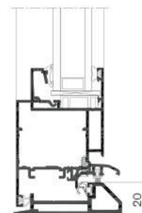
PORTE-FENÊTRE SEUIL DE 20 MM
