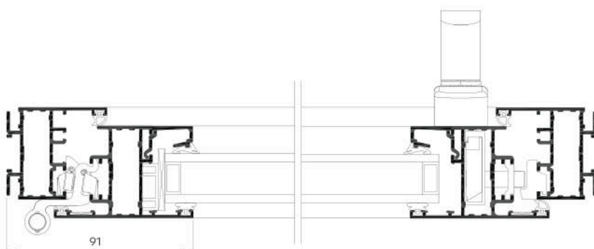
FENÊTRE 1 VANTAIL OUVRANT À L'ANGLAISE
