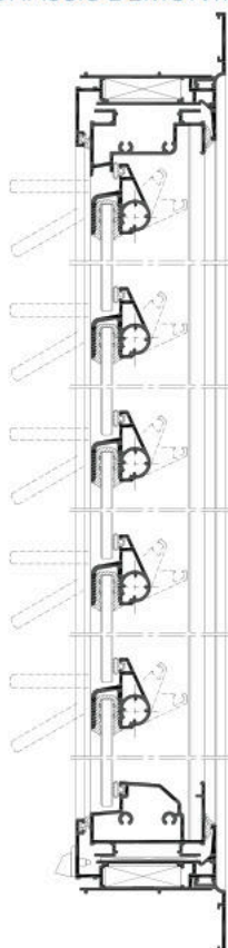
CHÂSSIS DÉMONTABLE
